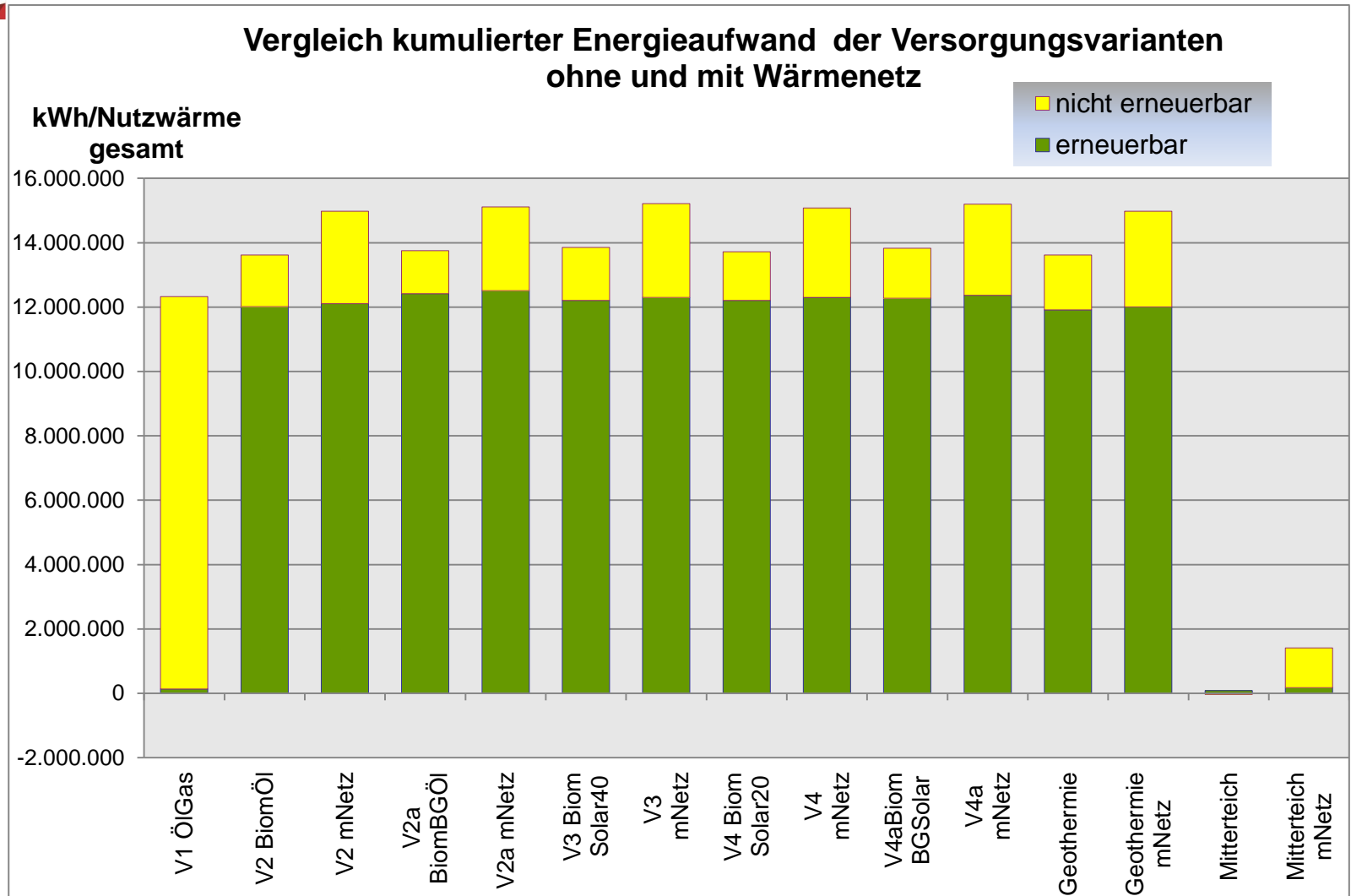
Abbildung: Vergleich kumulierter Energieaufwand der Wärmeversorgungsvarianten V1-4, 6 und Mitterteich ohne und mit Wärmenetz - eigene Darstellung auf Basis GEMIS
