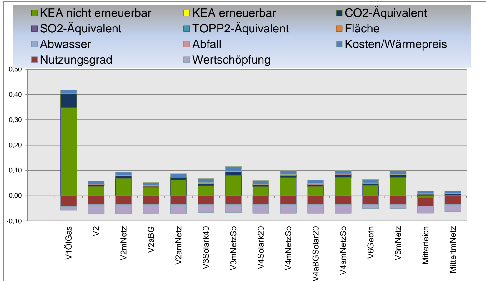
Abbildung: Ergebnis Vergleich Umweltauswirkungen der Wärmever- sorgungsvarianten ohne und mit Wärmenetz und Erdwärmespeicher – eigene Darstellung auf Basis GEMIS
